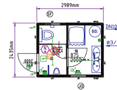
Bungalow sanitaire 10'
