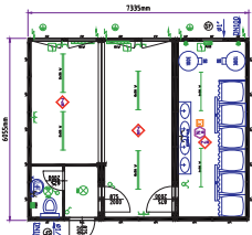
Ensemble de 3 bungalows bureaux et sanitaires
