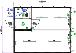
Ensemble de 2 bungalows bureaux et sanitaires
