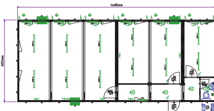
Ensemble de 6 bungalows bureaux et sanitaires
