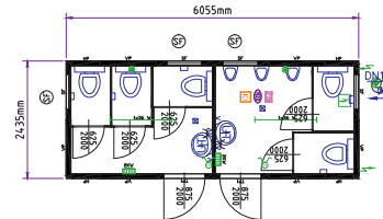
Bungalow WC 20' hommes et femmes
